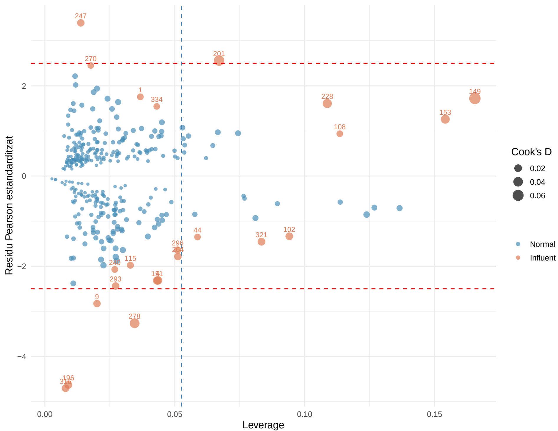
Leverage vs Residus de Pearson estandarditzats
